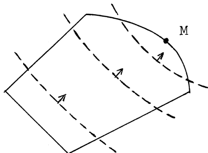
Figuur 3.11 Gebied convex Kriterium functie concaaf
